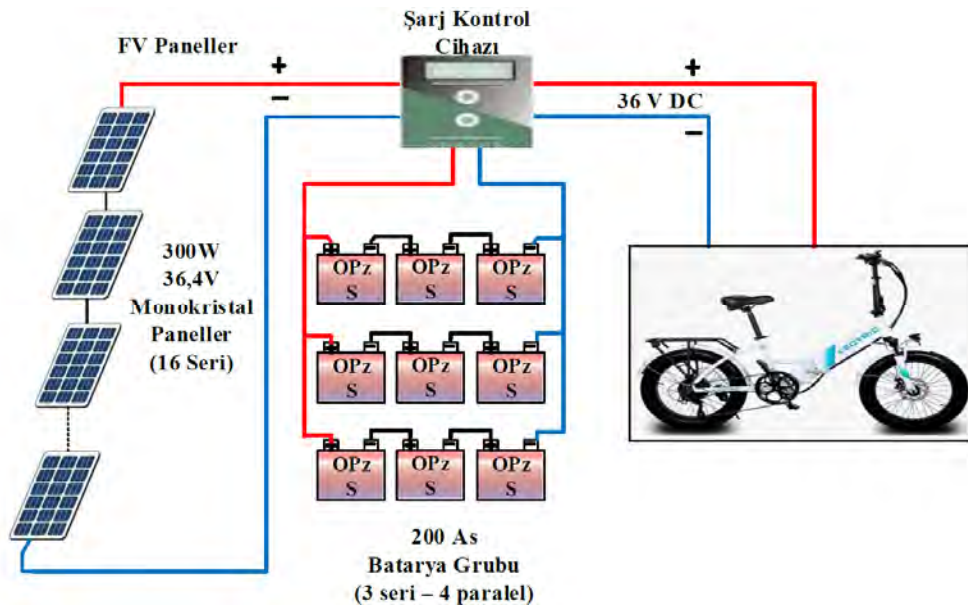
Şekil 5. E-bisiklet şarj sistemi blok şeması
